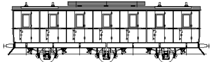
Ref A801 : 3 ème classe C7 17001 à 17416 (7 compartiments sans WC) Les deux faces sont identiques
