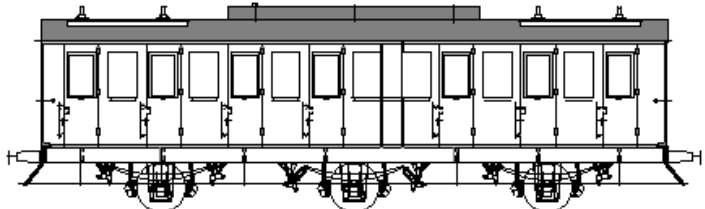
Ref A802 : 3 ème classe C7t 13588 à 13850 (7 compartiments avec WC) Face côté ouloir
