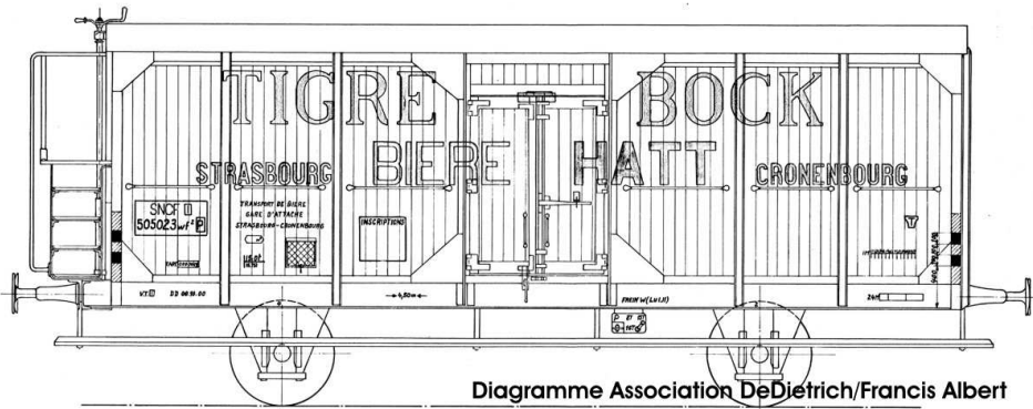
K245 caisse renforcée, plateforme de guérite haute, marchepieds sur toute la longueur boîtes d'essieux et tampons AL, déco Tigre-Bock AL/SNCF38
